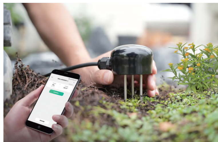
智能土壤温湿度计 产品型号：160101 电压/功率：24V dc / 1W 通信方式：PLC 防护等级：IP68 外形尺寸：60*80*102mm
