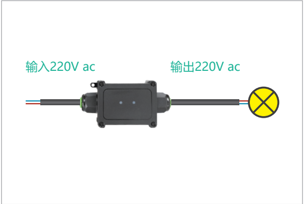
智能220V开关盒 产品型号：121201 电压/电流：220V ac / 最大5A 通信方式：PLC 防护等级：IP65 外形尺寸：66*126*41mm
