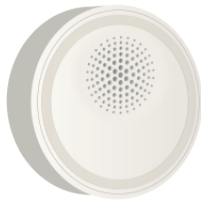
智能门铃 产品型号：130701 电压/功率：220V ac / 2W 通信方式：Wi-Fi 防护等级：无 外形尺寸：Φ81*48mm
